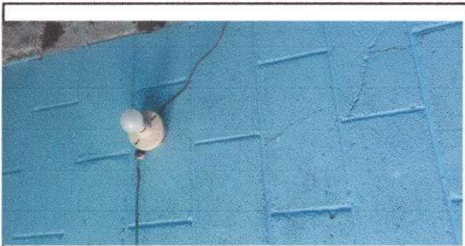
Foto 11: Reparación de cableado eléctrico, un total de 70 ML.
